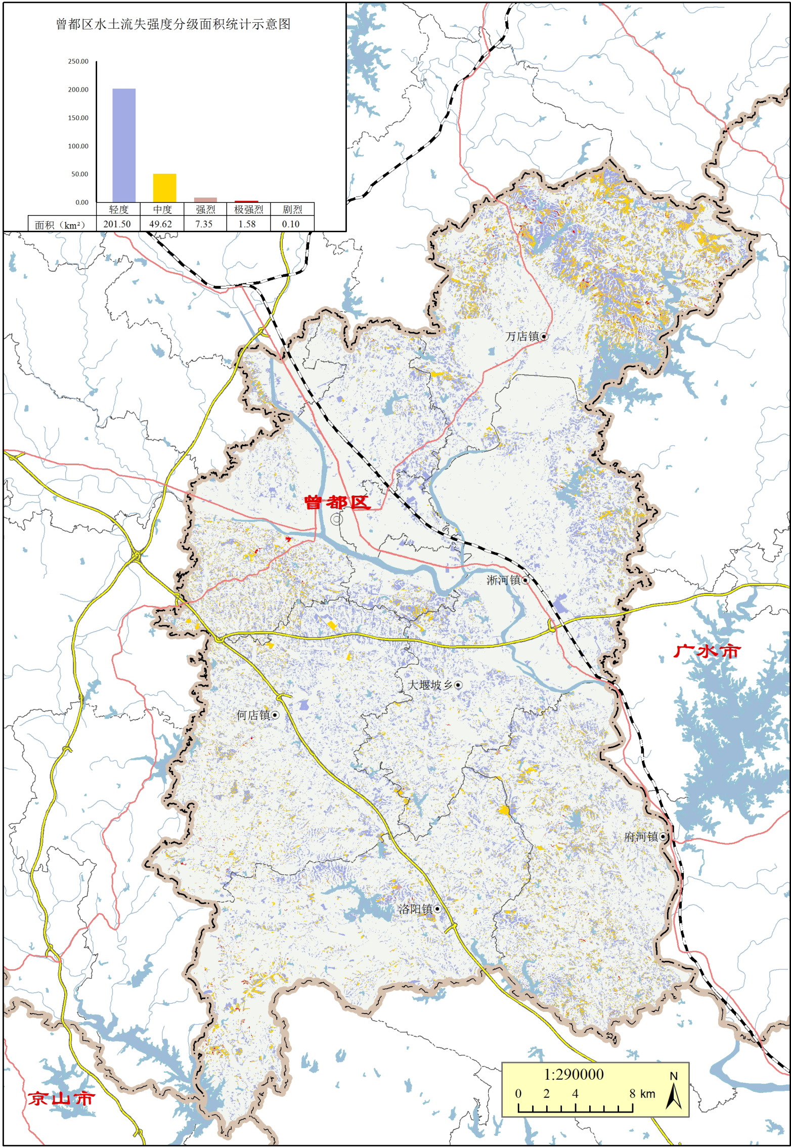
2022 年曾都区水土流失现状图
