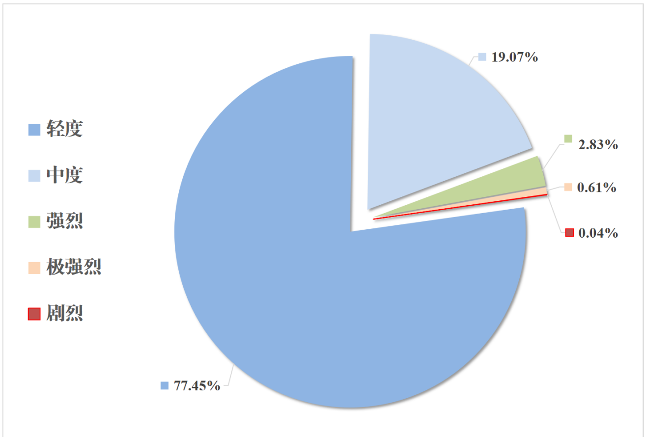
曾都区水土流失强度组成图
