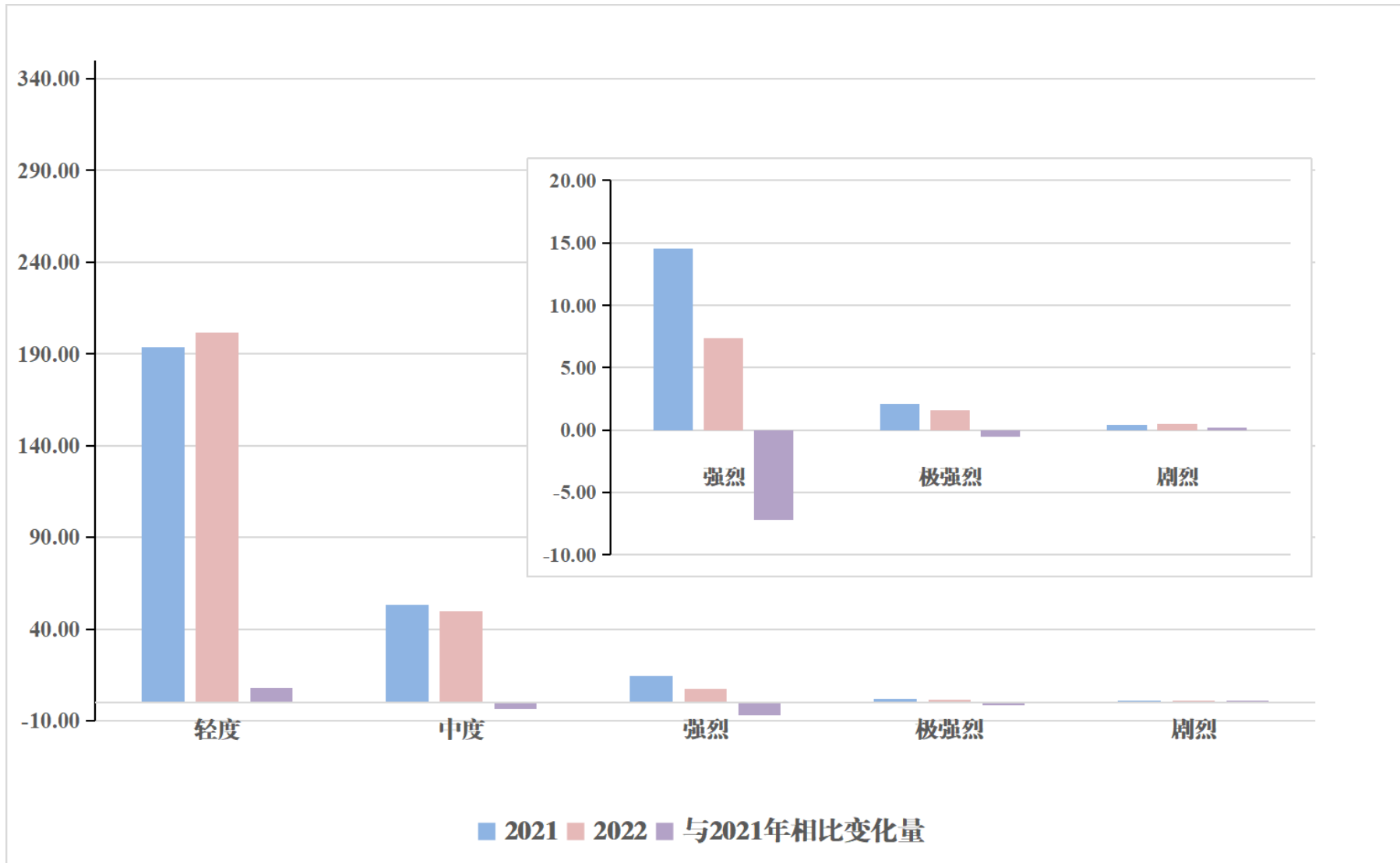
曾都区水土流失面积动态变化柱状图
